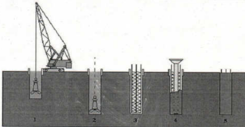
Figura 3. Construcción de pilotes TREMIE en zonas con nivel freático alto. Fuente: Procedimiento de construcción de cimentaciones y estructuras de contención. Yepes V (2020)
