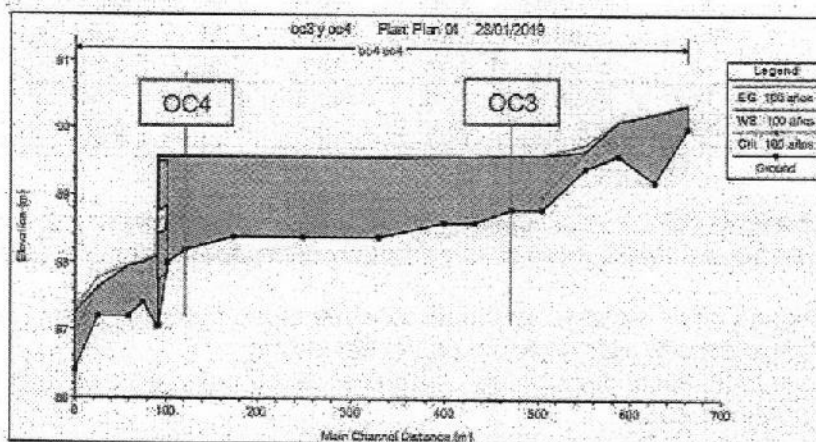
Figura 30 Perfiles del flujo en el cauce de la cuenca OC3 y OC4.
