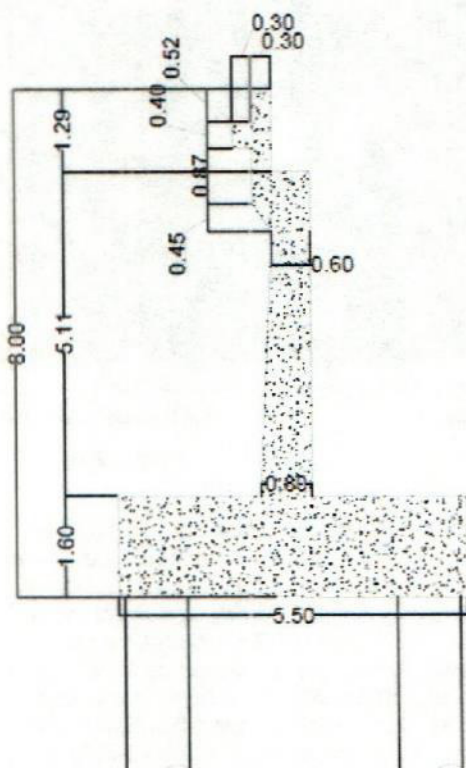
Figura 3. Dimensiones estribo puente. Fuente: Plano estructural solicitante
