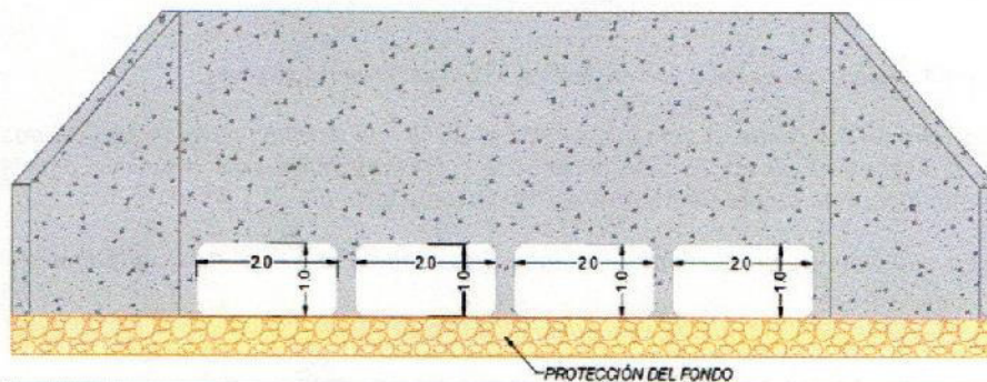
Figura 2. Esquema de la obra propuesta para K05+155.
