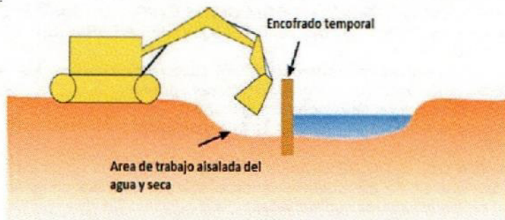
Figura 5. Aislamiento parcial con encofrado. Fuente: Adaptado de Engineering in the water environment. Good Practice SEPA 2009
