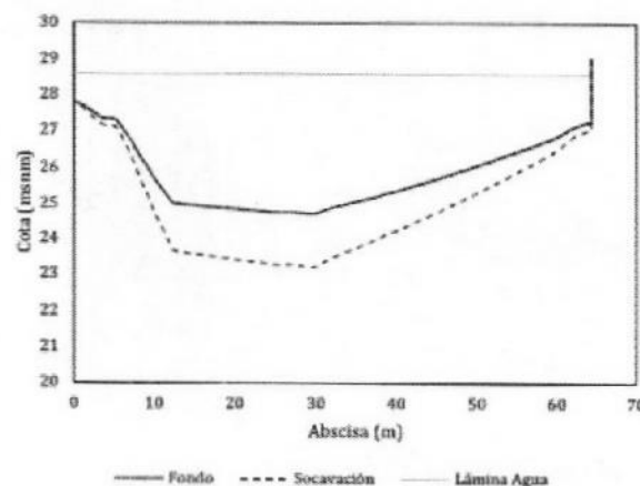
Figura 14. Perfil de socavación en el río Fundación para el periodo de retorno de 100 años.
