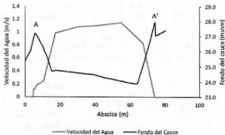
Figura 9. Perfil de velocidades para la sección A-A'. Caudal con periodo de retorno de 50 años.
