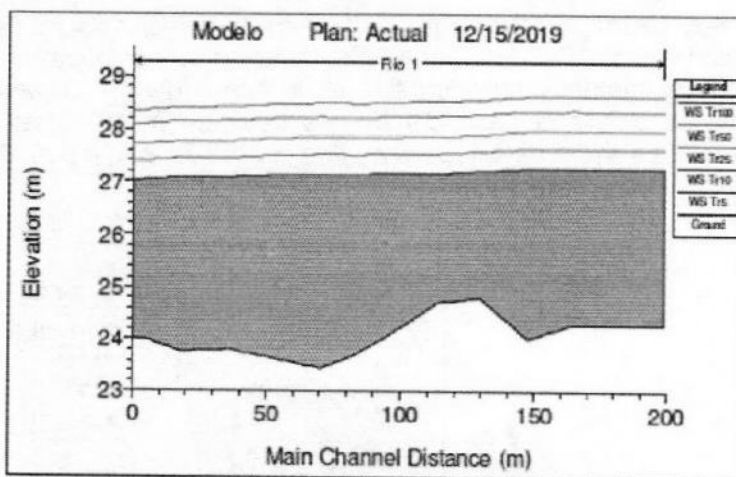
Figura 8. Corte longitudinal con los perfiles de agua para periodos de retorno de 10, 25, 50 y 100 años.
