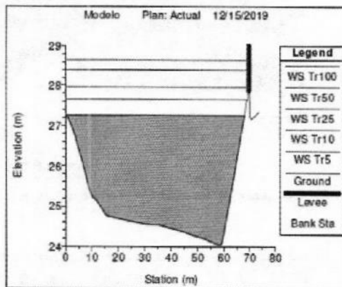
Figura 11. Lámina de agua esperada para distintos periodos de retorno sobre el río Fundación. Corte A-A'.
